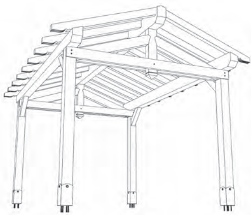
schema a due acque
